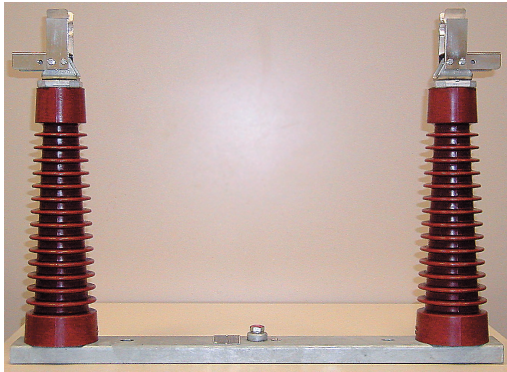
Abb./Fig. 10 HH-Sicherungsträger Innenraum HV fuse-base indoor 36 kV
