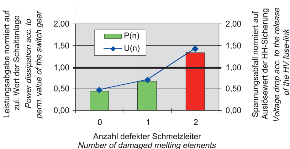
Abb./Fig. 8: Überwachte Leistungsabgabe/Controlled power dissipation
