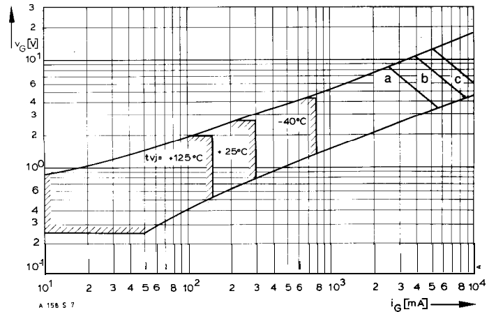
Bild/Fig. 19 Steuercharakteristik mit Zündbereichen/Gate Characteristic with triggering areas V_G = f(i_G) , V_0 = 12 V
