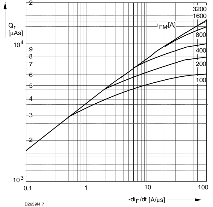
Bild / Fig. 6 Sperrverzögerungsladung / Recovered charge Q_r = f(-di_F/dt) t_{vj} = t_{vjmax} ; V_R \leq 0,5 V_{RRM} ; V_{RM} = 0,8 V_{RRM} Beschaltung / Snubber: C = 1,5 \mu F ; R = 2,7 \Omega Parameter: Durchlaßstrom / Forward current i_{FM}
