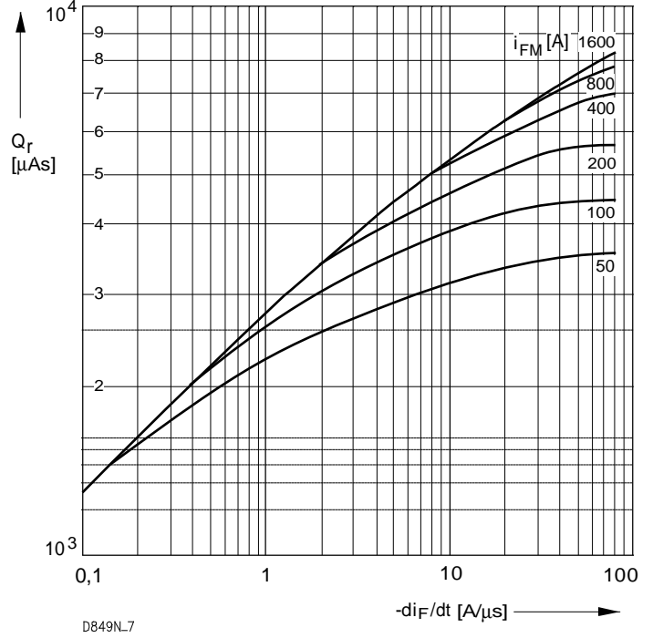
Bild / Fig. 6 Sperrverzögerungsladung / Recovered charge Q_r = Q - dI/dt t_{vj} = t_{vjmax} ; v_R \leq 0,5 V_{RRM} ; V_{RM} = 0,8 V_{RRM} Beschaltung / Snubber: C = 1 \mu F ; R = 3,9 \Omega Parameter: Durchlaßstrom / Forward current i_{FM}
