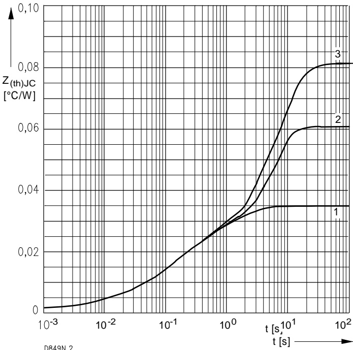
Analytische Elemente des transienten Wärmewiderstandes Z_{thJC} für DC Analytical elements of transient thermal impedance Z_{thJC} for DC
