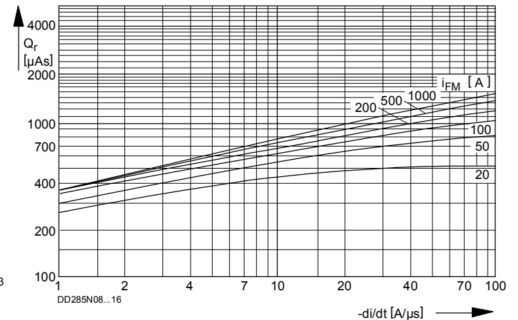
Bild/Fig. 6 Sperrverzögerungsladung / Recovered charge Q_r = f(-di/dt) t_{vj} = t_{vj \max} \cdot v_R \leq 0,5 V_{RRM} ; v_{RM} = 0,8 V_{RRM} Parameter: Durchlaßstrom / Forward current i_{FM}
