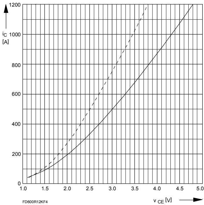
Bild/Fig. 1 Kollektor-Emitter-Spannung im Sättigungsbereich (typisch) Collector-emitter-voltage in saturation region (typical) V_{GE} = 15\text{V} ----- T_{vj} = 25^\circ\text{C} ——— T_{vj} = 125^\circ\text{C}
