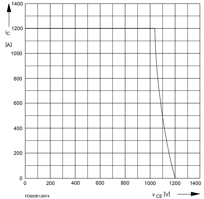
Bild/Fig. 4 Rückwärts-Arbeitsbereich Reverse biased safe operating area t_{vj} = 125^\circ\text{C} , v_{LE} = v_{LR} = 15\text{V} , R_G = 1,6\text{W}
