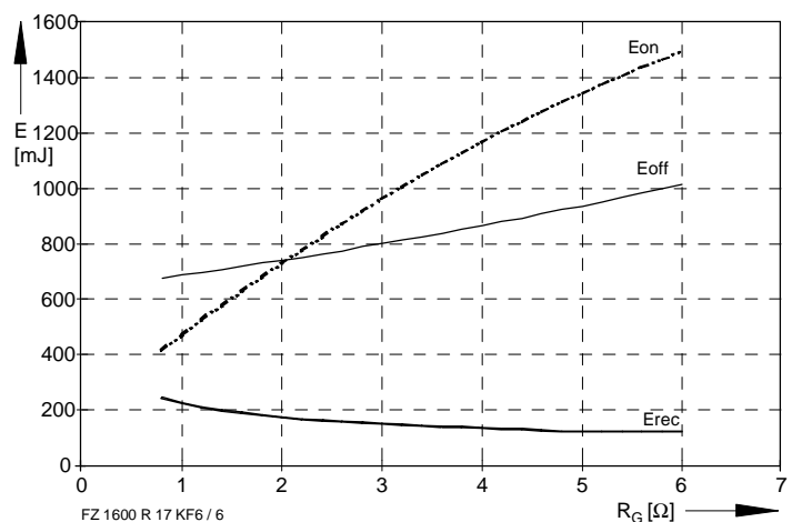
Bild / Fig. 6 Schaltverluste (typisch) / Switching losses (typical) E_{on} = f(R_G) , E_{off} = f(R_G) , E_{rec} = f(R_G) I_C = 1600A , V_{CE} = 900V , T_j = 125^\circ C
