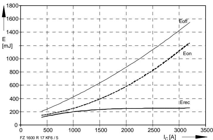
Bild / Fig. 5 Schaltverluste (typisch) / Switching losses (typical) E_{on} = f(I_C) , E_{off} = f(I_C) , E_{rec} = f(I_C) R_{gon} = R_{goff} = 0,9\Omega , V_{CE} = 900V , T_j = 125^\circ C
