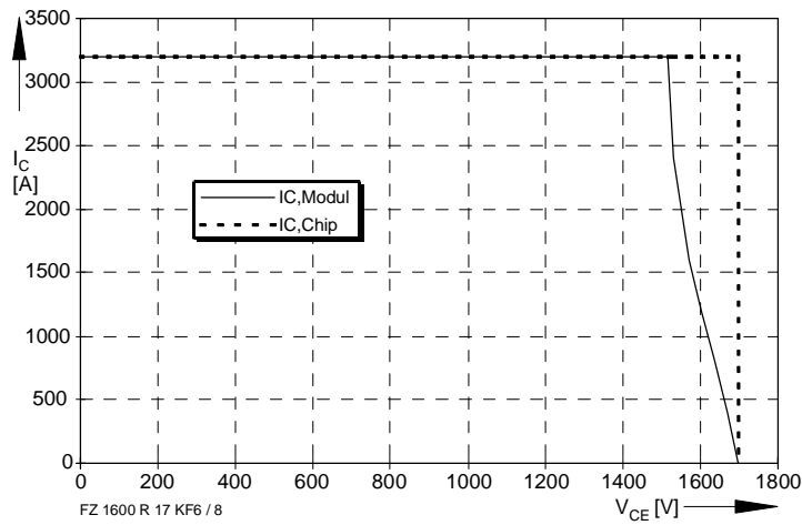
Bild / Fig. 8 Sicherer Arbeitsbereich (RBSOA) / Reverse bias safe operation area (RBSOA) R_g = 0,9\Omega , T_{vj} = 125^\circ\text{C}
