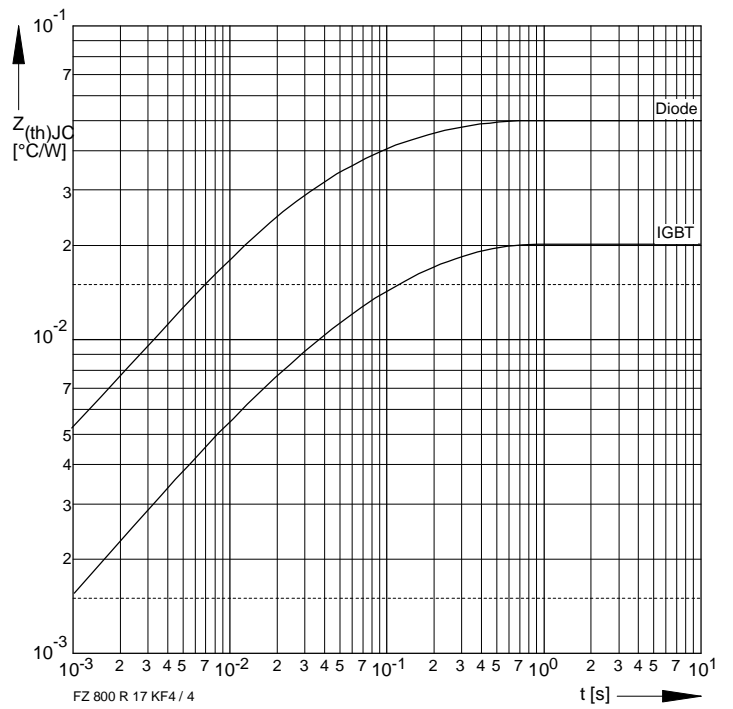
Bild / Fig. 4 Transienter innerer Wärmewiderstand (DC) / Transient thermal impedance (DC)
