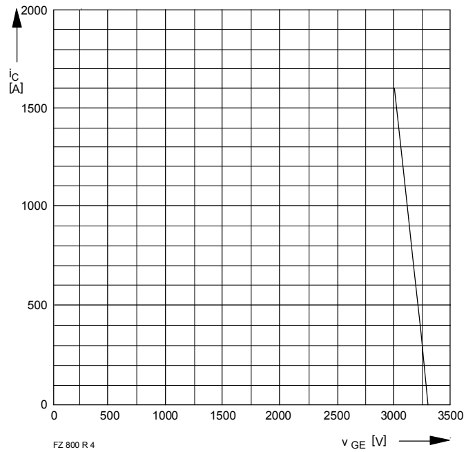
Bild/Fig. 4 Rückwärts-Arbeitsbereich Reverse biased safe operating area t_{vj} = 125 \text{ }^\circ\text{C} , v_{LF} = v_{LR} = 15 \text{ V} , R_{GF} = 2,7 \text{ } \Omega , R_{GR} = 5,1 \text{ } \Omega C_{GE} = 150 \text{ nF} , dv_{CE}/dt \leq 3000 \text{ V}/\mu\text{s}
