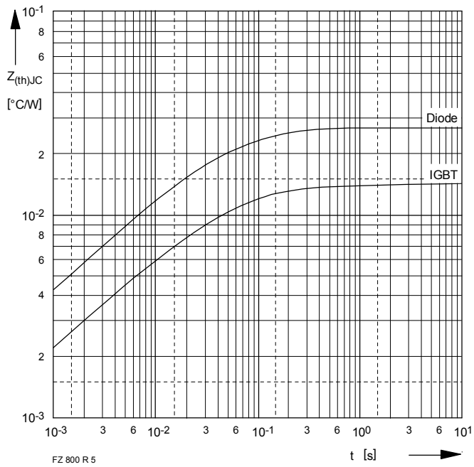
FZ 800 R 5 Bild/Fig. 5 Transienter innerer Wärmewiderstand (DC) Transient thermal impedance (DC)
