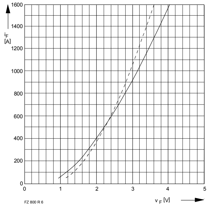
FZ 800 R 6 Bild/Fig. 6 Durchlaßkennlinie der Inversdiode (typisch) Forward characteristic of the inverse diode (typical) ..... t_{vj} = 25^{\circ}C — t_{vj} = 125^{\circ}C
