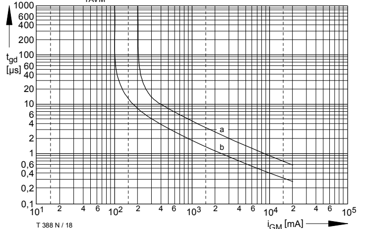
Bild / Fig. 18 Zündverzögerung / Gate controlled delay time t_{gd} = f(i_{GM}) t_{vj} = 25\text{ °C} , di_G/dt = i_{GM}/1\mu\text{s} a - Maximaler Verlauf / Limiting characteristic b - Typischer Verlauf / Typical characteristic
