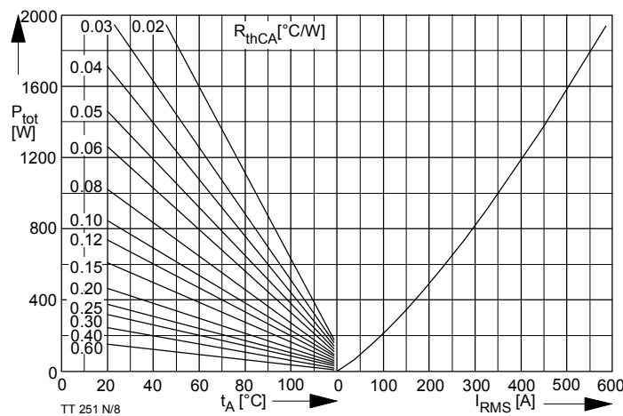
Bild / Fig. 8 W3C - Dreiphasen-Wechselwegschaltung / Three-phase inverse parallel circuit Höchstzulässiger Effektivstrom je Phase / Maximum rated RMS current per phase I_{RMS} Gesamtverlustleistung der Schaltung / Total power dissipation of the circuit P_{tot} Parameter: Wärmewiderstand zwischen den Gehäusen und Umgebung / thermal resistance case to ambient R_{thCA}
